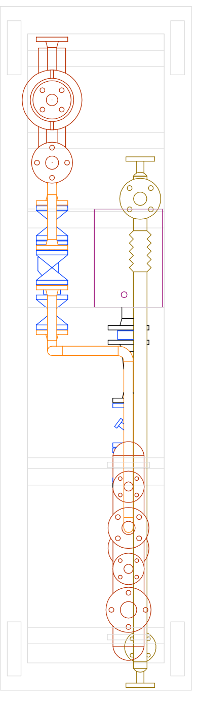
Réseau retour condensat 16b vers Chaudière
